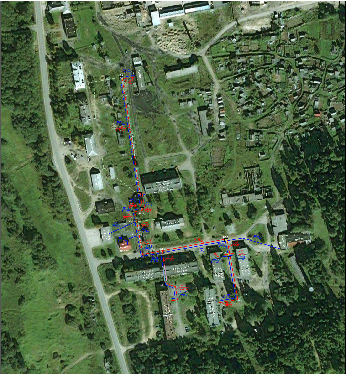
Схема теплоснабжения п.Подборовье Масштаб 1:50000
